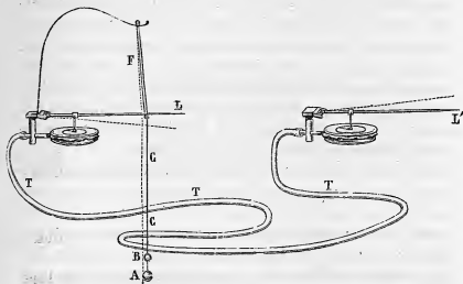
Fig. 102. — Transmission d'un mouvement de va-et-vient au moyen d'un simple de traction.
